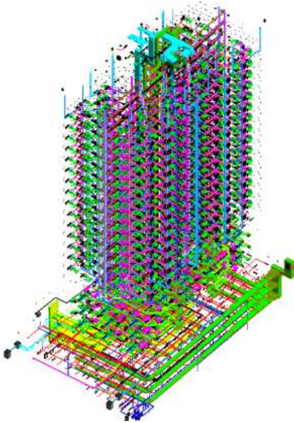
MÔ HÌNH REVIT HỆ CƠ
